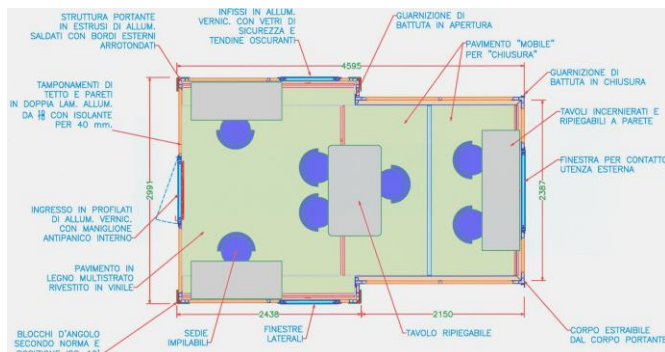
Sezione in pianta in posizione operativa
