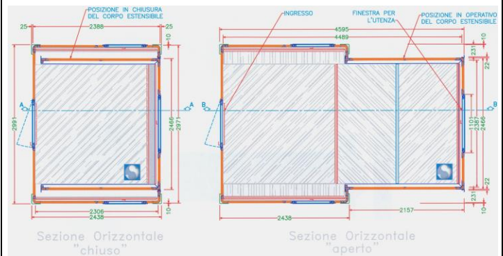
Vista/disegno in sezione orizzontale "chiuso"
