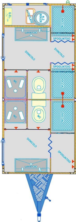
Vista/disegno in pianta del complessivo
