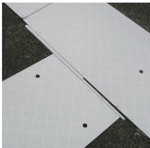
Particolare di cerniere, incastri e forature di fissaggio
